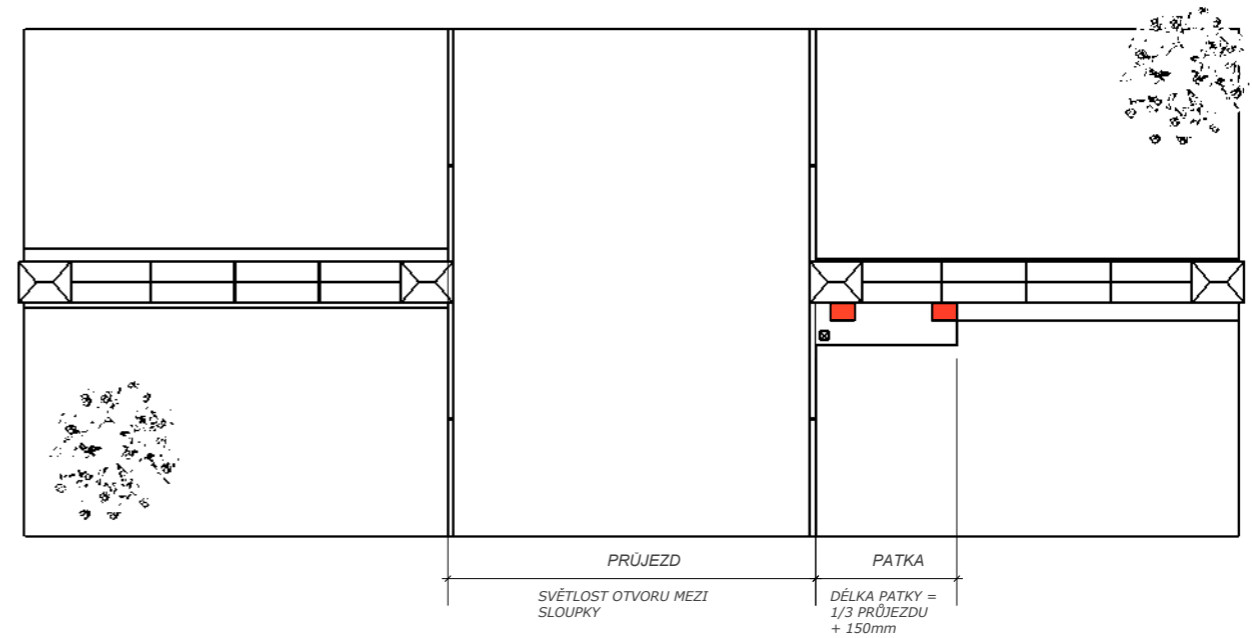
A PŮDORYS
