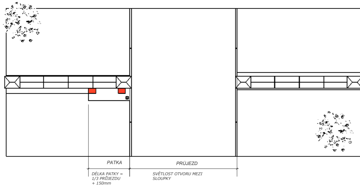
A PŮDORYS
