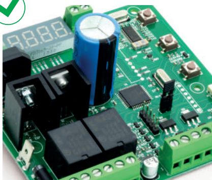
S řídicí jednotkou NET324N
